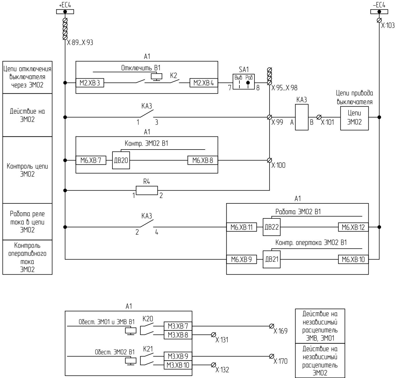
Цепи ЭМ02
